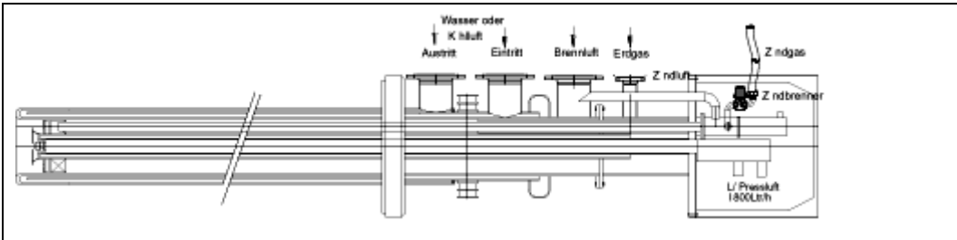
Öl-Gas-Lanzenbrenner mit Wasser oder Luftkühlung oder Feuerfestisolierung. Leistung bis 60 MW. (Andere Leistungen auf Anfrage)
