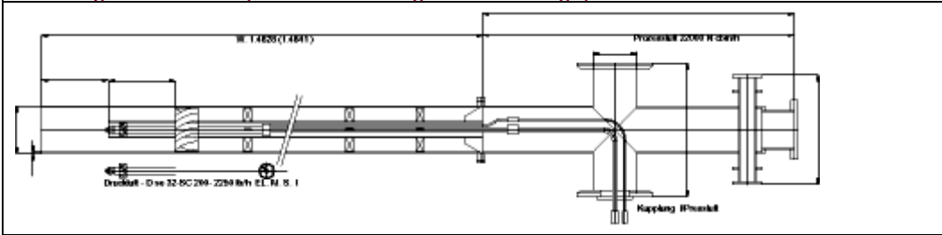
Lanzenbrenner Als Schmelz- und Warmhaltebrenner in der Kupferindustrie
