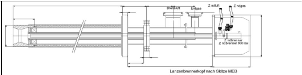
Temperbrenner 0,8 MW
